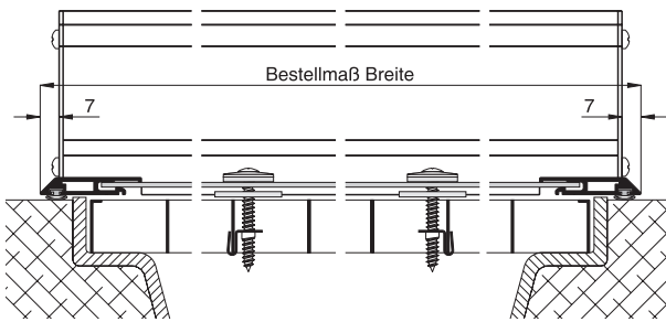
Vertikalschnitt Breite (Vorderansicht)
