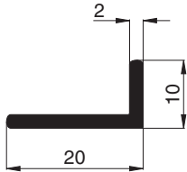
10 90 35 Winkelprofil 20/10/2
