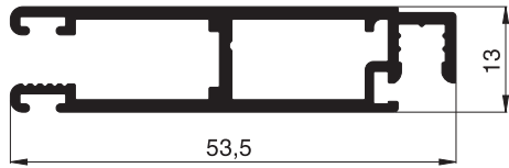
10 48 02 Schiebeflügelprofil
