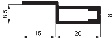
10 23 13 Montagerahmenprofil
