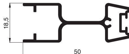
10 45 05 Griffleiste
