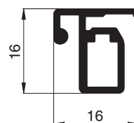
10 33 46 Lichtschachtdeckungsprofil
