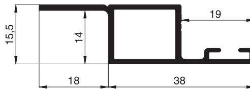
10 35 24 Montagerahmenprofil
