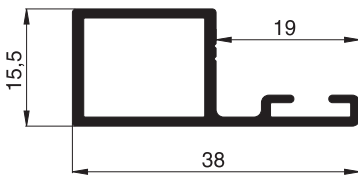
10 35 21 Montagerahmenprofil
