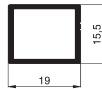
10 35 22 Montagerahmenprofil
