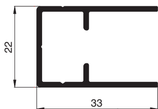
10 45 04 Rahmenprofil
